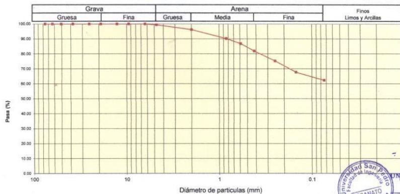
CURVA GRANULOMÉTRICA
