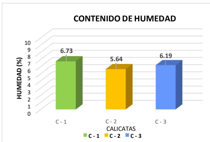
Figura N°1: Contenido de humedad del suelo en el Barrio Tacllan Bajo-Huaraz
