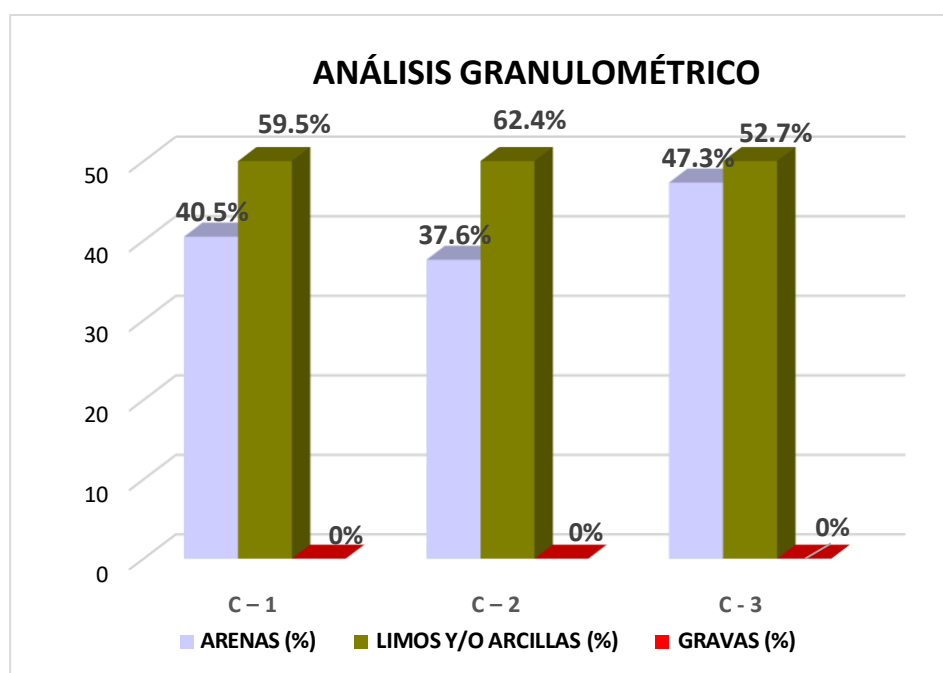
Figura N°2: Análisis granulométrico del suelo en el Barrio Tacllan Bajo-Huaraz
