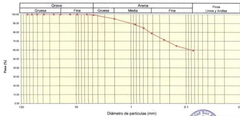
CURVA GRANULOMÉTRICA
