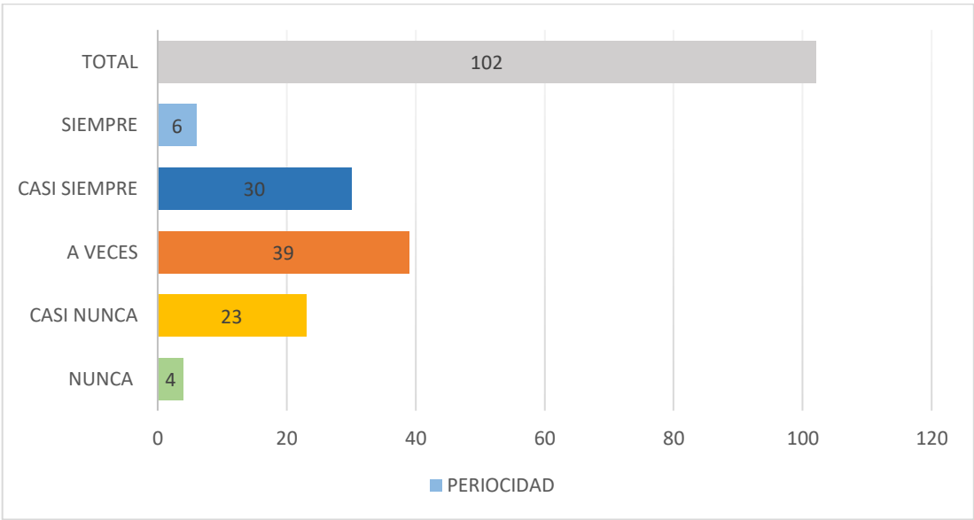
figura 1. Categoría de estimación para la magnitud identificación apreciadas por los usufructuarios de la Botica Perfumería Piura, 2025.
