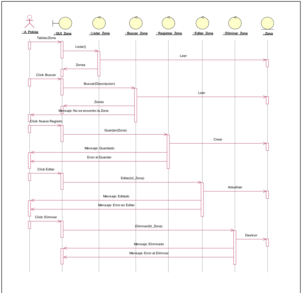
Figura 20: Diagrama de Secuencia de Registro de Zona
