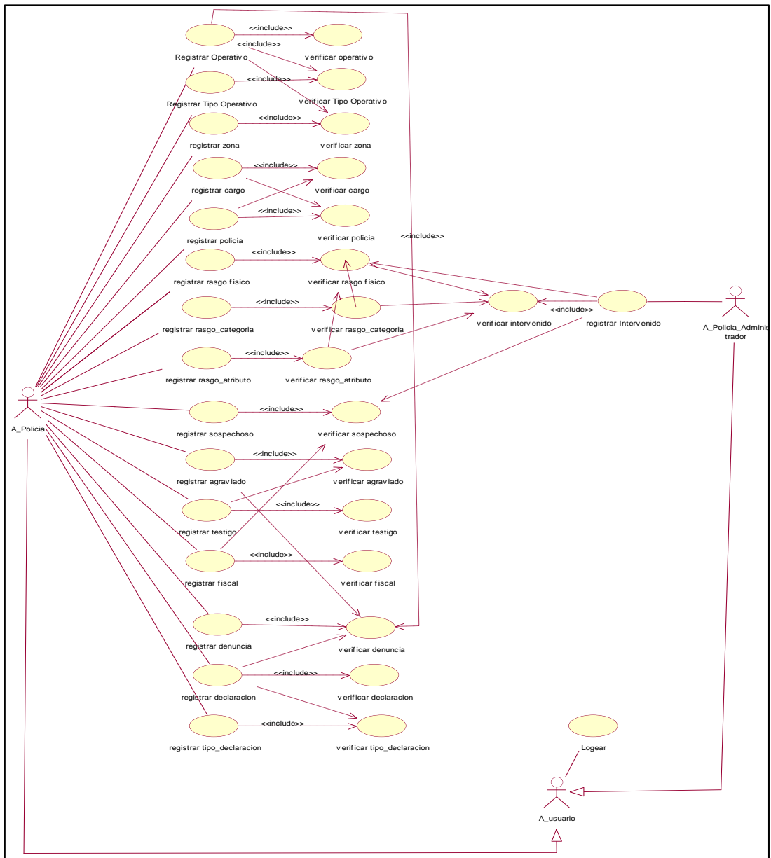
Figura 15: Modelo de caso de uso
