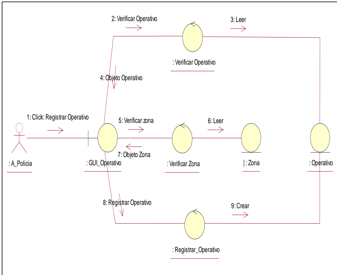
Figura 17: Diagrama de colaboración – Registrar Operativo
