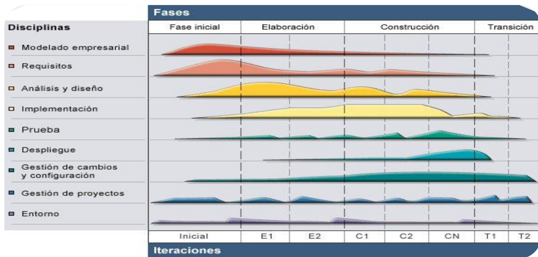
Figura 5: Fases de la metodología RUP
