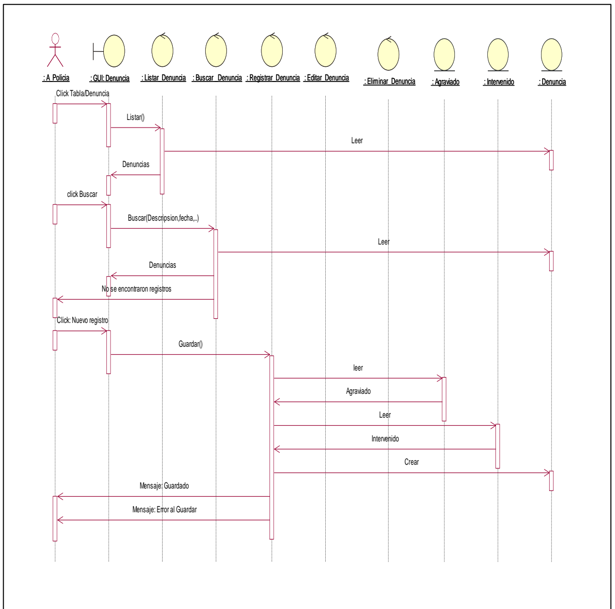
Figura 22: Diagrama de Secuencia de Registro de Denuncia
