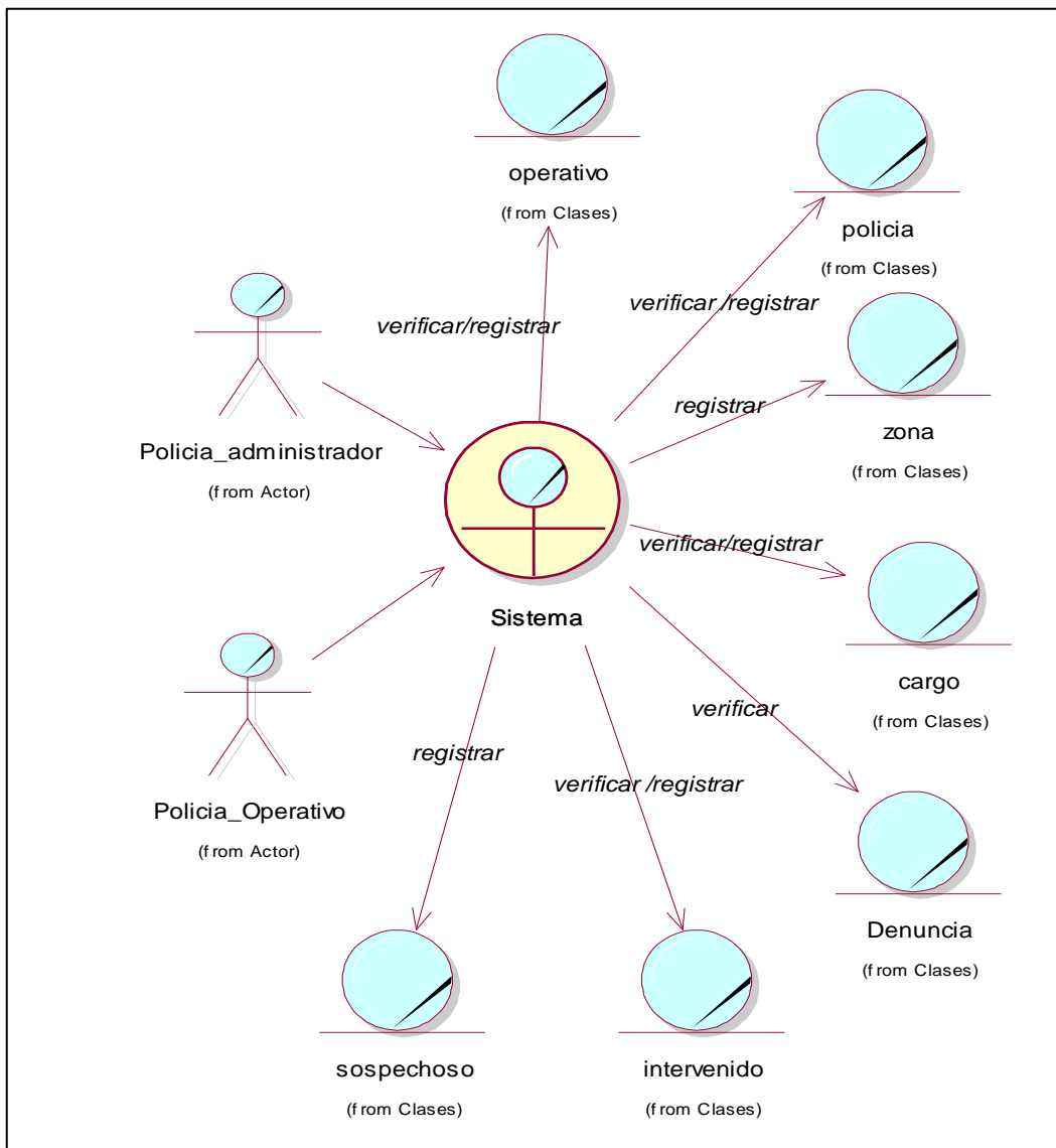
Figura 9: Modelo de objetos de negocio – Gestión de Operativo
