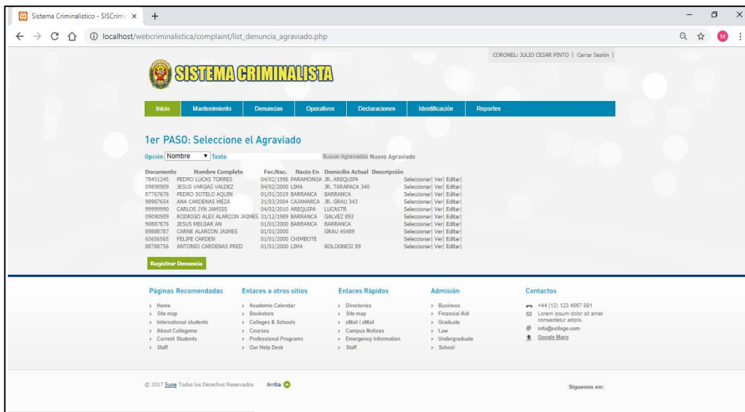
Figura 29: Interfaz gráfica de Gestión de denuncia - Selección del Agravado
