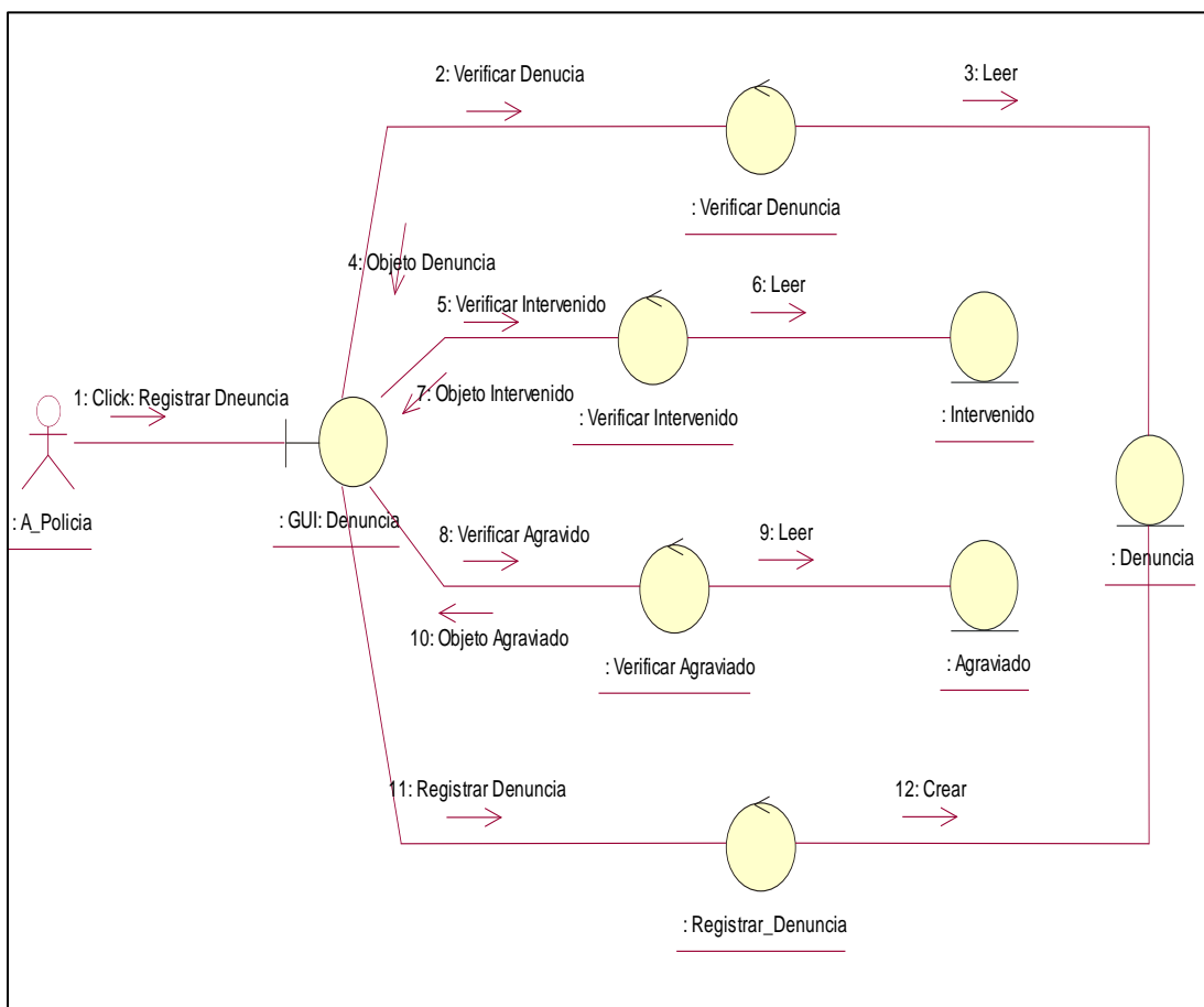
Figura 16: Diagrama de colaboración – Registrar Denuncia
