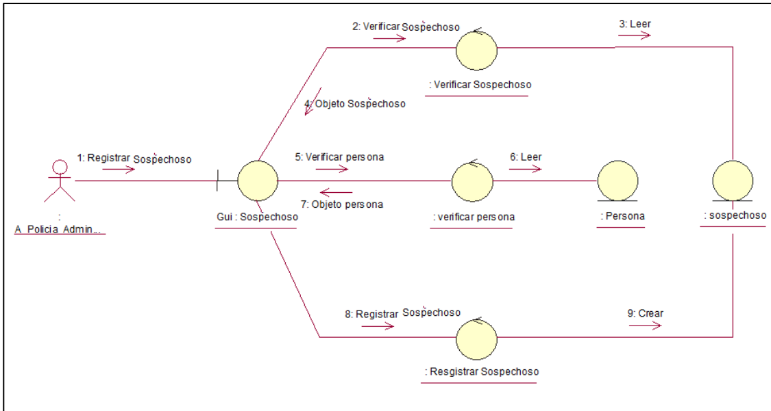
Figura 18: Diagrama de colaboración – Registrar Sospechoso
