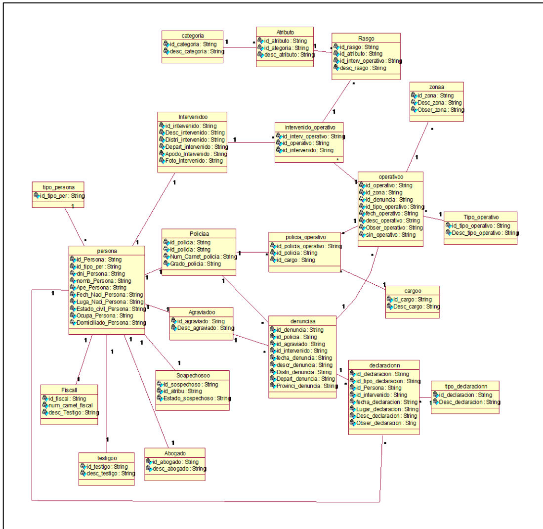
Figura 19: Diagrama de Clases de análisis
