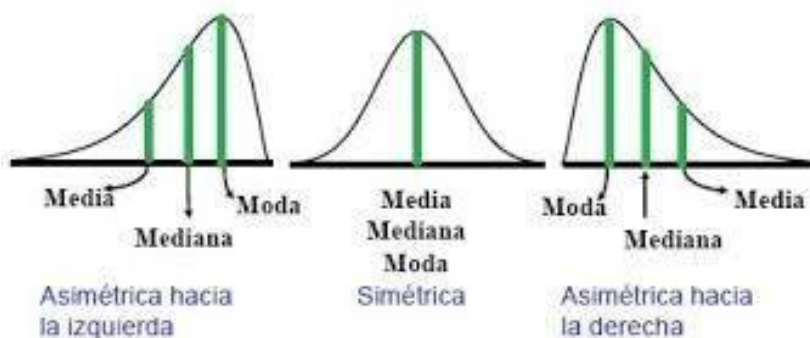
Figura 3 Tipos de campanas de Gauss, Coeficiente de Fisher Fuente: Fundamentos básicos de estadística, Cecilia Salazar y Santiago del Castillo 2018p 77
